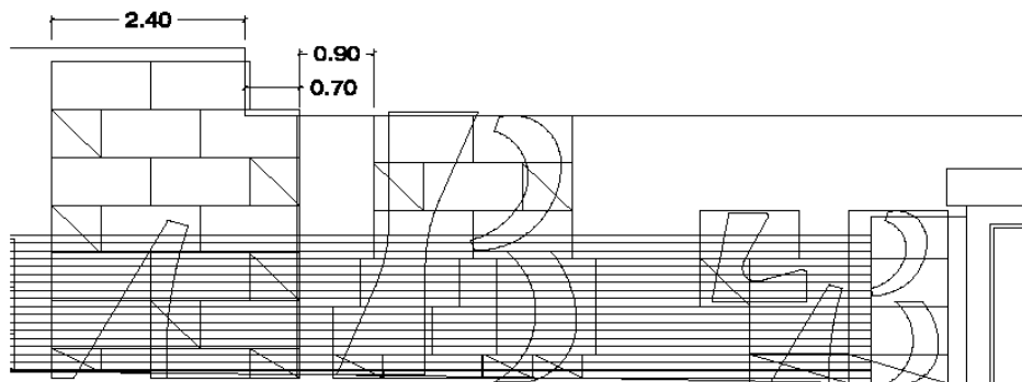
Alçat mur Farell · Símbols (lletres i números) · Detall (Especejament de planxes XPS)
